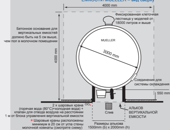
ГАБАРИТНЫЕ РАЗМЕРЫ ВЕРТИКАЛЬНОЙ ЕМКОСТИ MUELLER – вид сверху
