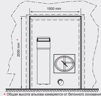
ГАБАРИТНЫЕ РАЗМЕРЫ АЛЬКОВА ВЕРТИКАЛЬНЫХ ЕМКОСТЕЙ MUELLER вид спереди
